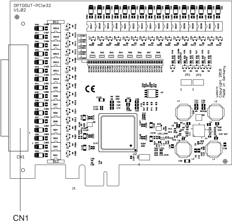
CN1: Optokoppler-Ausgänge OUT00...OUT31
