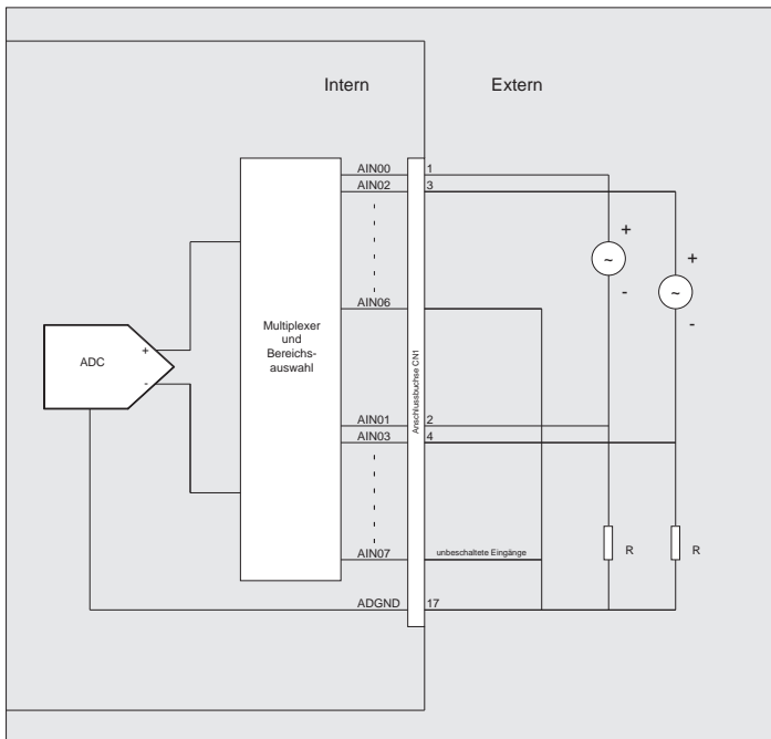
Grafik 10.5 Beschaltung der AD-Eingänge (differentiell)
