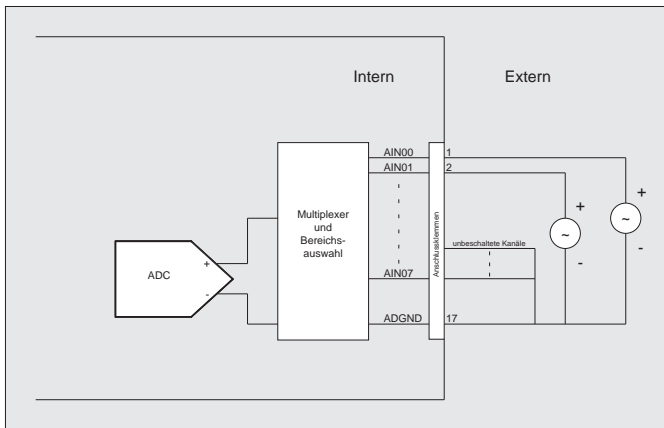
Grafik 15.4 Beschaltung der AD-Eingänge (Single-ended)
