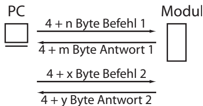
Grafik 12 Kommunikationsmodell
