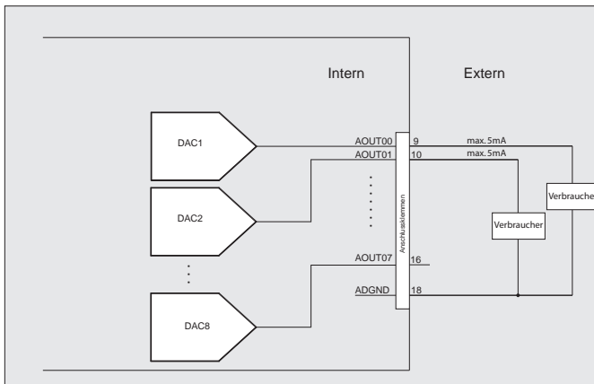
Grafik 15.3 Beschaltung der DA-Ausgänge
