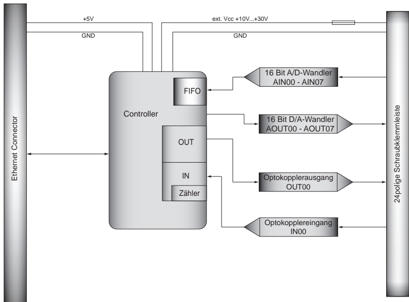
Grafik 3.2 Blockschahtbild EXDUL-584S
