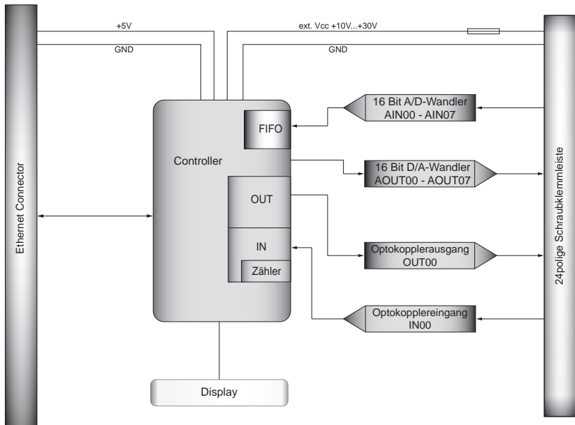
Grafik 3.1 Blockschahtbild EXDUL-584E
