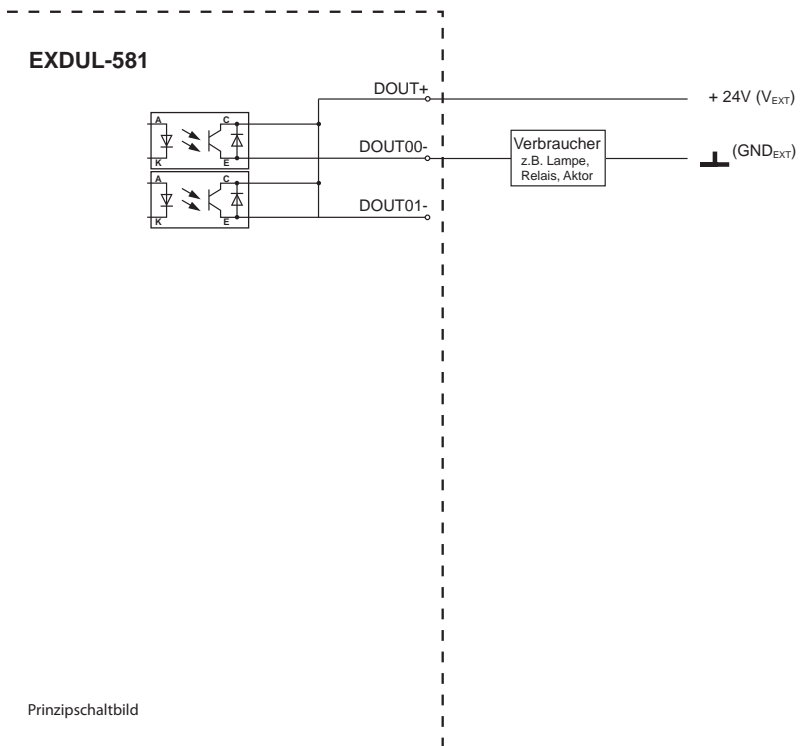
Grafik 14.2 Beschaltung der Optokoppler-Ausgänge
