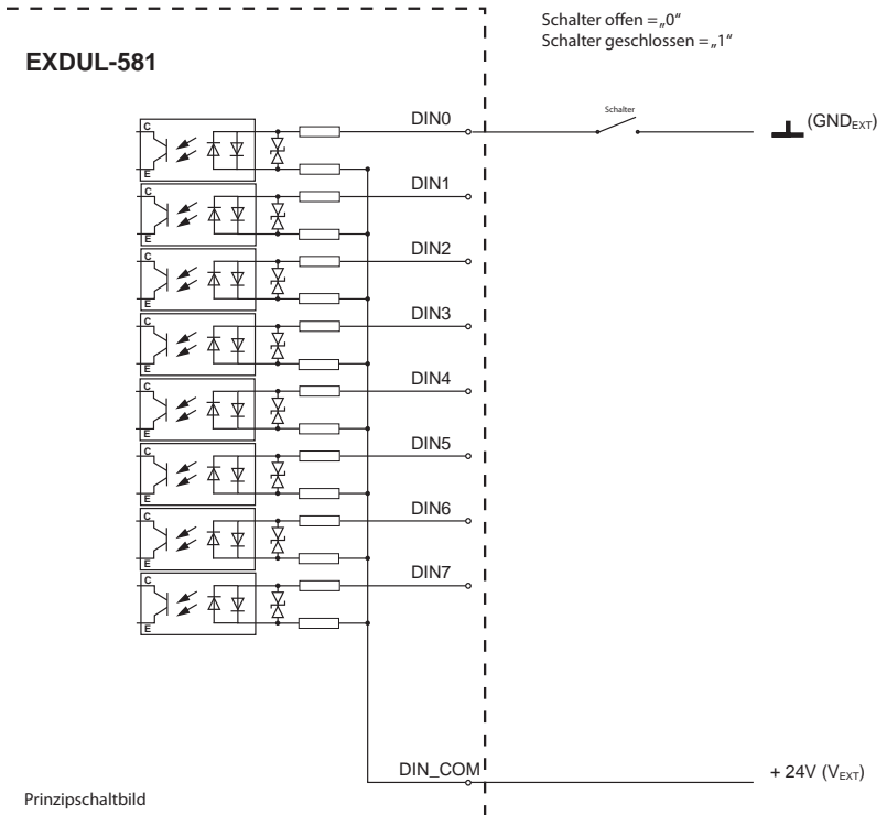
Graphik 14.1.2 Beschaltung der Optokopplereingänge revers
