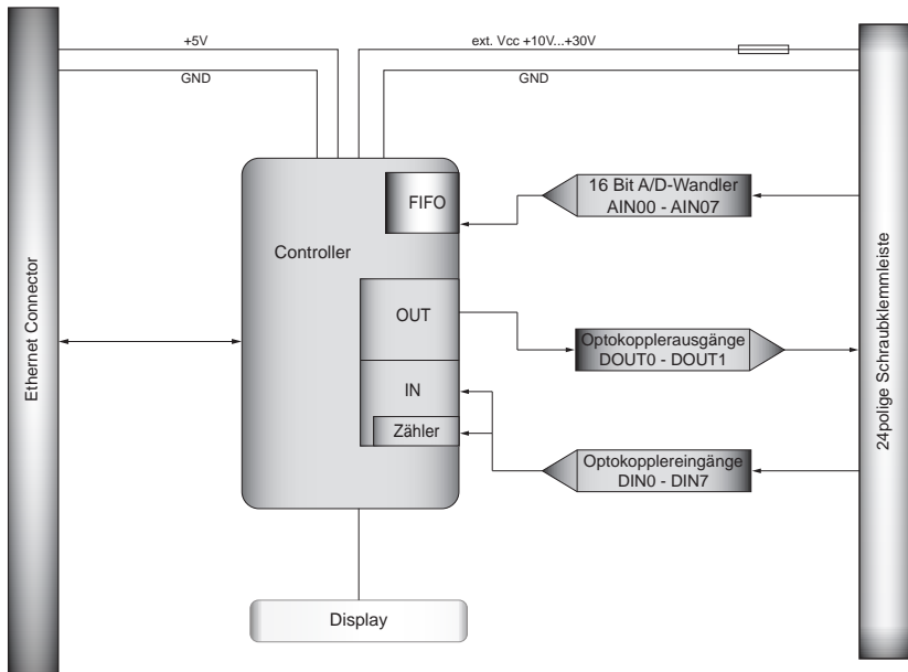
Grafik 3.1 Blockschaubild EXDUL-581E
