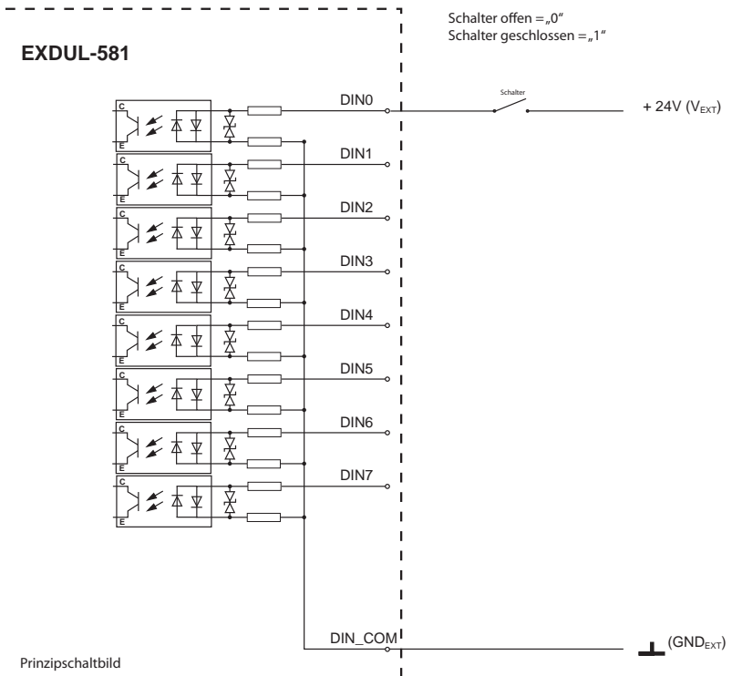
Grafik 14.1.1 Beschaltung der Optokopplereingänge
