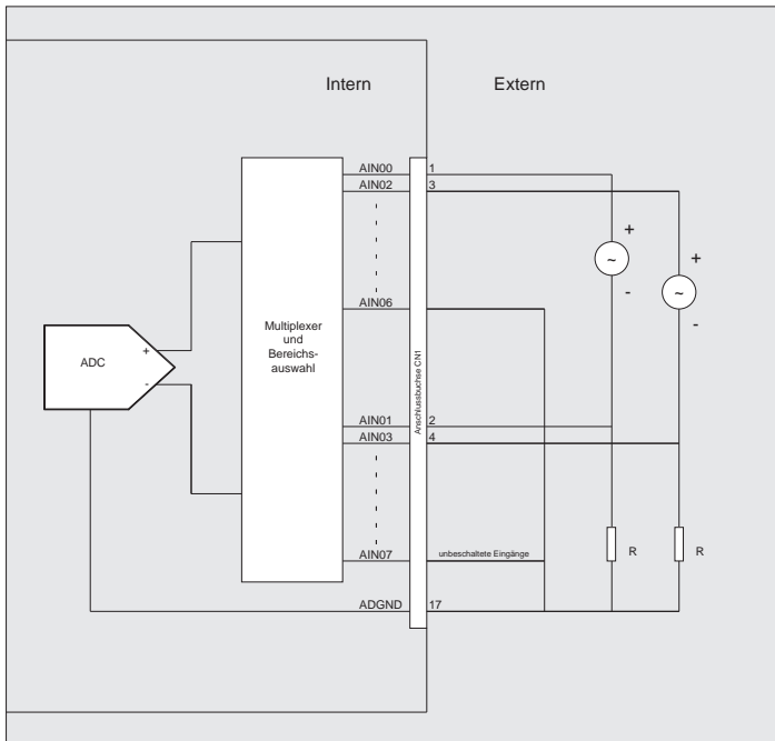
Grafik 14.4 Beschaltung der AD-Eingänge (differentiell)
